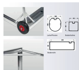
Netzbügel und Bodenrohr für Sandfüllung für Tor 125
