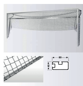
Bodenrahmen Nr. 194 für Tor 100 - bei Tortiefe 150cm - stabil - mit Netzschiene
