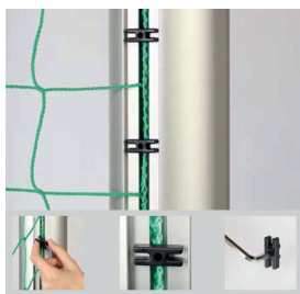
NETZRAHMEN H+ 555SL inkl. bei Tor 101 pro Tor
